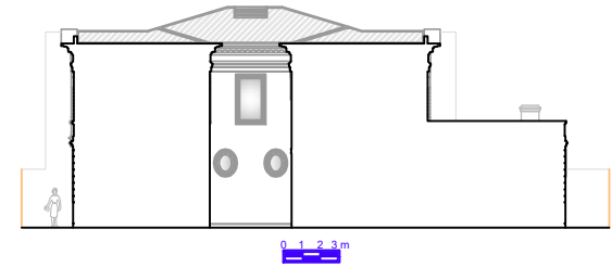
Elevation 04
